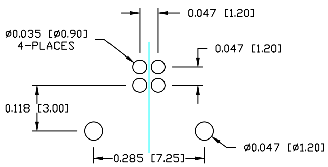
P.C.B LAYOUT
